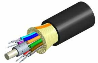
FO OM3 LazrSPEED®
